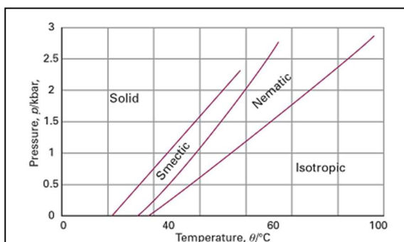
Abb. 4.4 Das Phasendiagramm des Flüssigkristalls Octylcyanobiphenyl (8CB, Abb. 4.5). Zwischen dem Kristall und der isotropen Flüssigkeit befinden sich zwei weitere, teilgeordnete Phasen. digitalfirst.bfwpub.com/qchem2e_impact_sections/impact_14_2.html Basierend auf: R. Shashidhar, G. Venkatesh, J. de Physique Colloque , 40 , C3 (1979).
