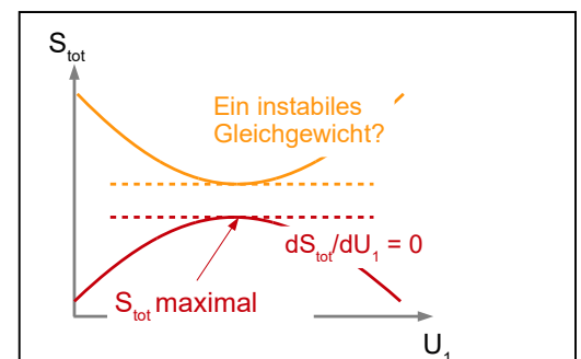
Abb. 5.15 Für ein stabiles thermisches Gleichgewicht ist die Gesamt-Entropie maximal. Die Tangente an das Maximum ist horizontal ( dS_{\text{tot}}/dU_1 = 0 ).
