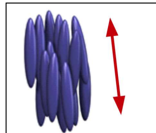
Abb. 4.6 In der nematischen Phase haben die Moleküle eine gemeinsame Vorzugsrichtung. Es gibt aber keinen „Pfeil“. „Oben“ und „Unten“ sind gleichwertig. en.wikipedia.org/wiki/Liquid_crystal
