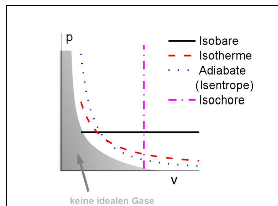
Abb. 3.2 Ein pV-Diagramm. Man verzichtet auf eine dreidimensionale Darstellung und zeichnet stattdessen Linien zu konstanter Temperatur in die pV-Ebene ein. Hier ist nur eine solche Isotherme (rot, gestrichelt) dargestellt. Die „Isobare“ (eine Linie mit konstantem Druck) und die Isochore (eine Linie mit konstantem Volumen) sind in dieser Darstellung trivial. Die blau gepunktete Linie zeigt eine Adiabate. Eine Adiabate ergibt sich, wenn das Gas während der Zustandsänderung keine Wärme mit der Umgebung austauscht. Falls der Prozess als Gleichgewichtsprozess geführt ist, bleibt dann die Entropie konstant. Dann ist die Adiabate eine Isentropie.
