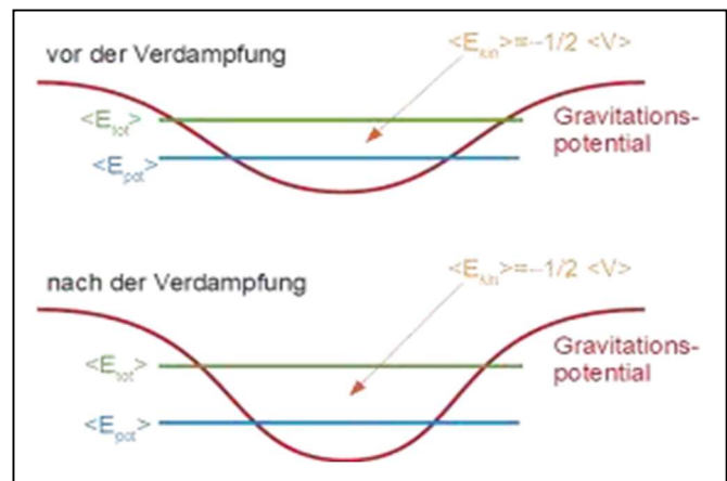
Abb. 5.13 Für selbst-gravitierende Wolken steigt beim Abdampfen von energiereichen Partikeln oder bei der Abstrahlung von Photonen die kinetische Energie (und damit auch die Temperatur).
