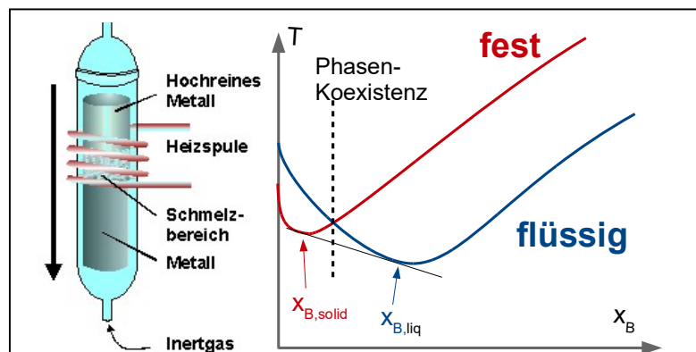
Abb. 9.29 Monokristallines Silizium wird durch Zonenschmelzen aufgereinigt. www.fbv.fh-frankfurt.de/mhwww/ach-vorlesung/Bilder/Si-hochrein.htm
