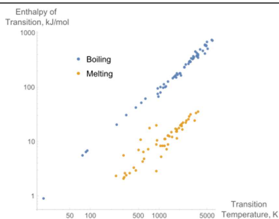
Abb. 7.17 Für das Schmelzen von Kristallen könnte man eine Regel ähnlich der Trouton-Regel aufstellen. Sie wäre aber als Regel deutlich schlechter. Die Schmelz-Entropien folgen dieser Regel nicht gut. en.wikipedia.org/wiki/Trouton's_rule
