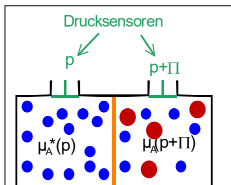
Abb. 9.17 Ein idealisierter Messaufbau für den osmotischen Druck. Das Volumen auf beiden Seiten der Membran ist konstant. Auf der Seite, die die Minoritätskomponente enthält, baut sich ein Überdruck auf.
