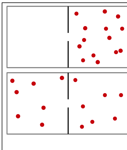
Abb. 2.2 Seien gegeben zwei Kammern, von denen die linke zu Beginn des Experiments leer sei. Wenn man ein kleines Loch öffnet, verteilen sich die Partikel gleichmäßig, weil sich dabei die Anzahl der möglichen Mikrozustände erhöht. Grundsätzlich könnten sich rein zufallsgesteuert alle Partikel wieder in der rechten Kammer versammeln, aber dies ist extrem unwahrscheinlich. Der Zustand mit gleicher Dichte und gleichem Druck auf beiden Seiten ( \Delta p \approx 0 ) ist ein thermodynamisches Gleichgewicht.
