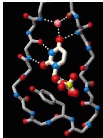
Abb. 9.14 Ein Beispiel für eine Wechselwirkung, wo das Prinzip „Gleiches löst Gleiches“ nicht zur Wirkung kommt. Man spricht von spezifischer Erkennung gemäß dem „Schlüssel-Schloss-Prinzip“. www.scripps.edu/~cliff/snap/pix.html
