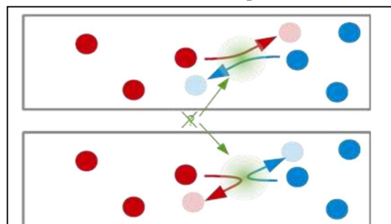
Abb. 9.5 Die Unterscheidbarkeit von Molekülen im Gas geht bei Stoßprozessen verloren. Die Frage, ob der Stoß gemäß dem oberen oder dem unteren Diagramm stattgefunden habe, kann niemals beantwortet werden. Wenn man zu Beginn alle Partikel links „rot“ nennt und alle Partikel rechts „blau“ nennt, dann ist gleichwohl die Farbe der Partikel nach den Stößen unbestimmt (blass gezeichnet).
