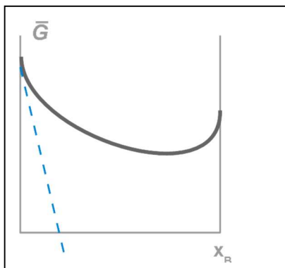
Abb. 9.28 Im thermodynamischen Grenzfall ( N \rightarrow \infty ) kann man eine Substanz B aus einer Mischung niemals vollständig entfernen, weil die Steigung der Funktion \bar{G}(x_B) bei x_B \rightarrow 0 unendlich wird.
