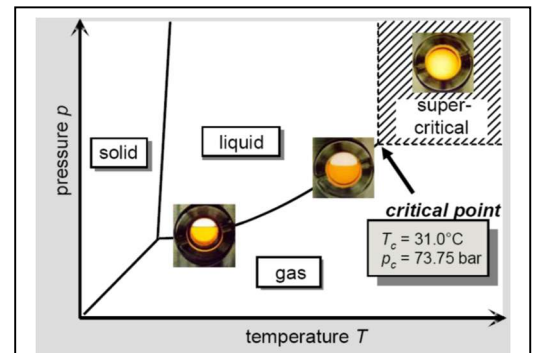
Abb. 3.10 Am kritischen Punkt verschwindet kontinuierlich der Unterschied zwischen Flüssigkeit und Dampf. www.gdch.de/strukturen/fg/leitner.pdf
