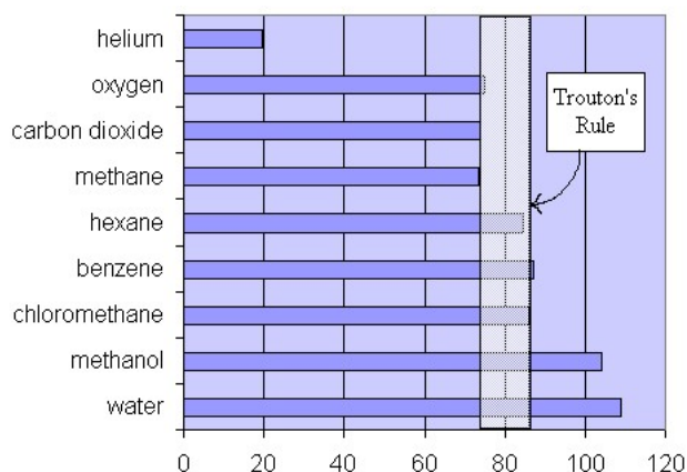
Abb. 7.16 Der Trouton-Quotient für eine Reihe von Flüssigkeiten www.chem.queensu.ca/people/faculty/mombourquette/FirstYrChem/slg/Troutons_rule.htm
