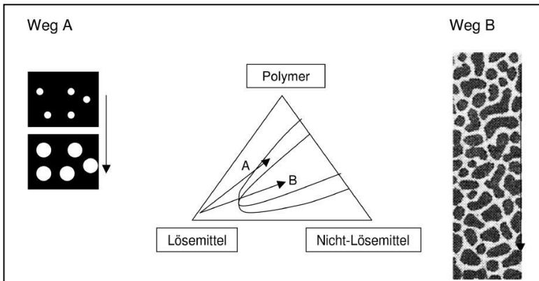
Abb. 1.3 Mechanismus der Phasentrennung während der Membranbildung.
